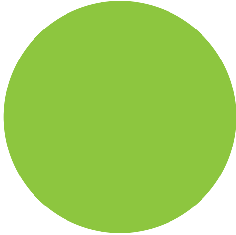
Atlantis
